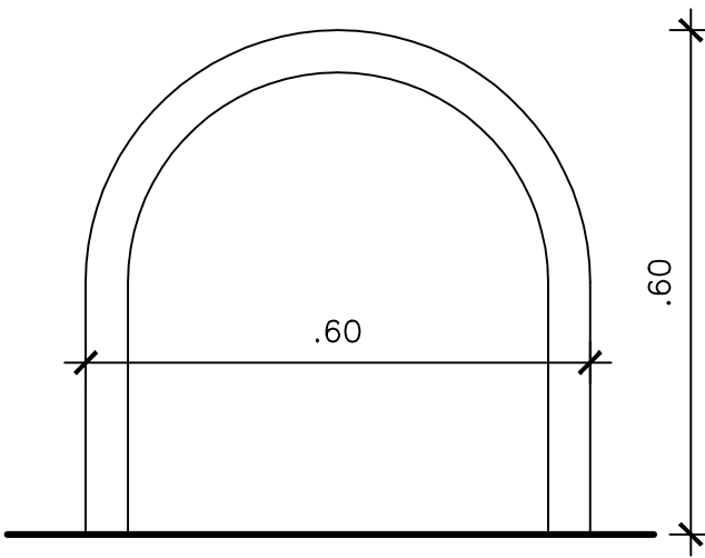
DETALHE Esc. 1:10
