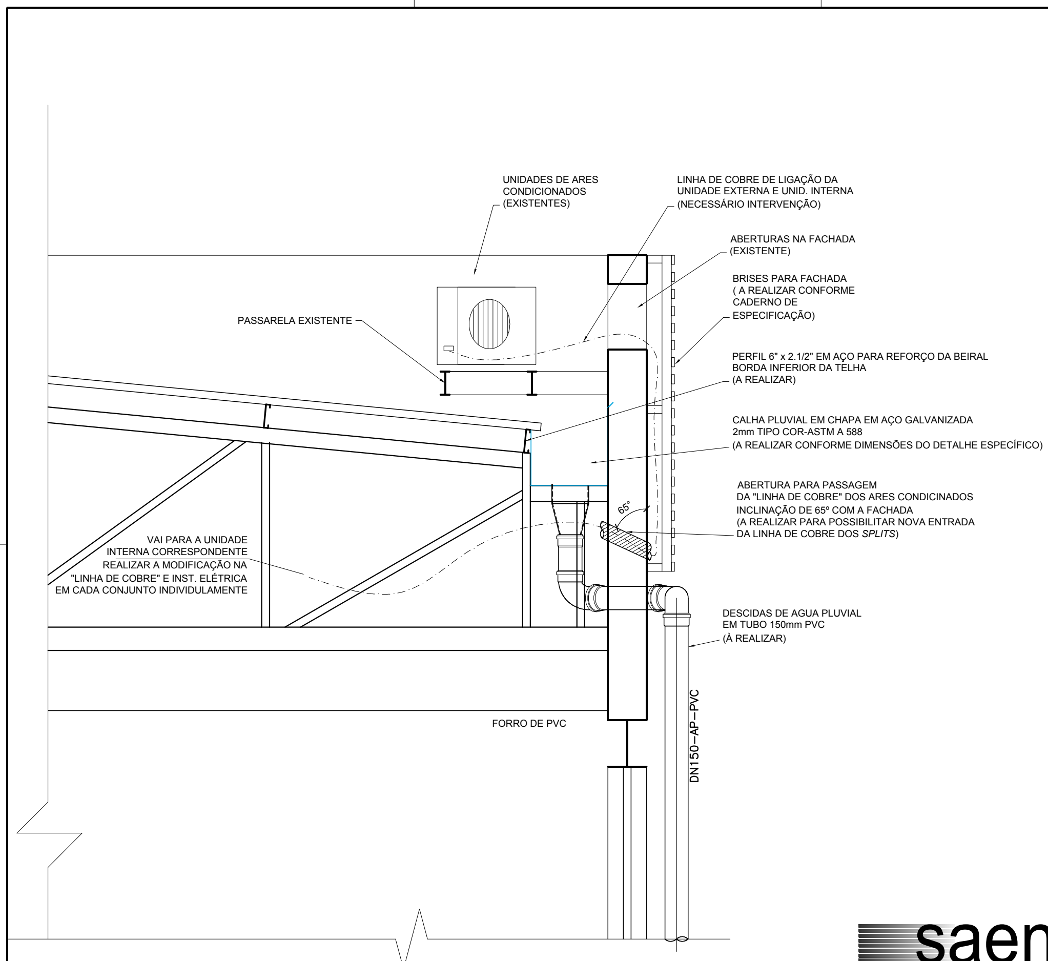
1 DETALHAMENTO INTERVENÇÃO DA LATIBANDA ESC.: 1/25
