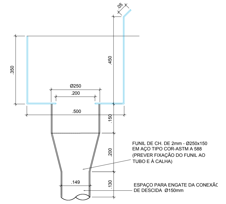
2 SEÇÃO DA CALHA PLUVIAL E DETALHE DO FUNIL DE CAPTAÇÃO ESC.: 1/10
