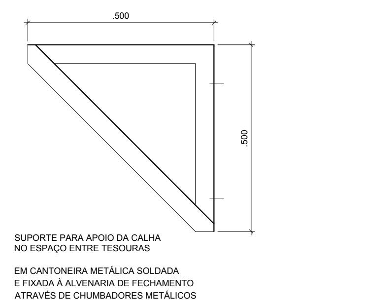
3 SUPORTE DA CALHA PLUVIAL ESC.: 1/10
