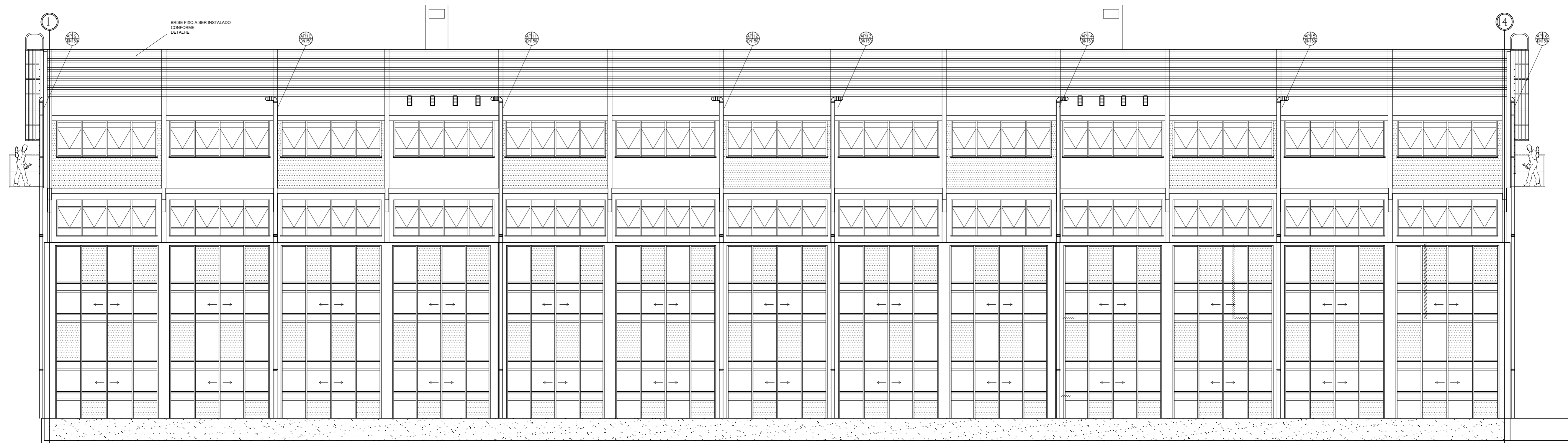
1 FACHADA SUL "MERCADO MUNICIPAL" ESC.: 1/100
