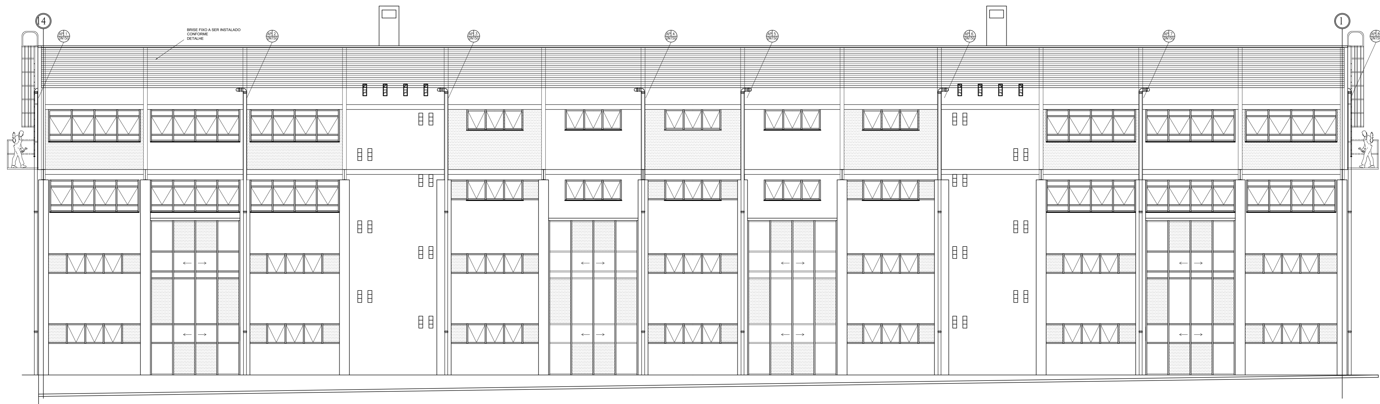
2 FACHADA NORTE "CSN" ESC.: 1/100
